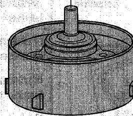
Bloc de fixation de l'axe du malaxeur (N° réf. ADA 29A115)
